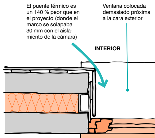
Figura 0.2 Ejemplo de puente térmico. 2
